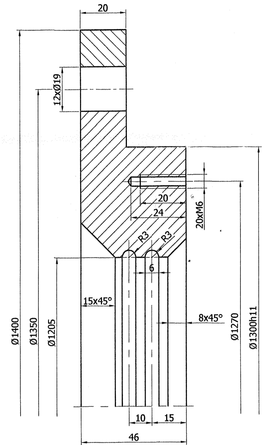
Szczegół "a" (1:1)
